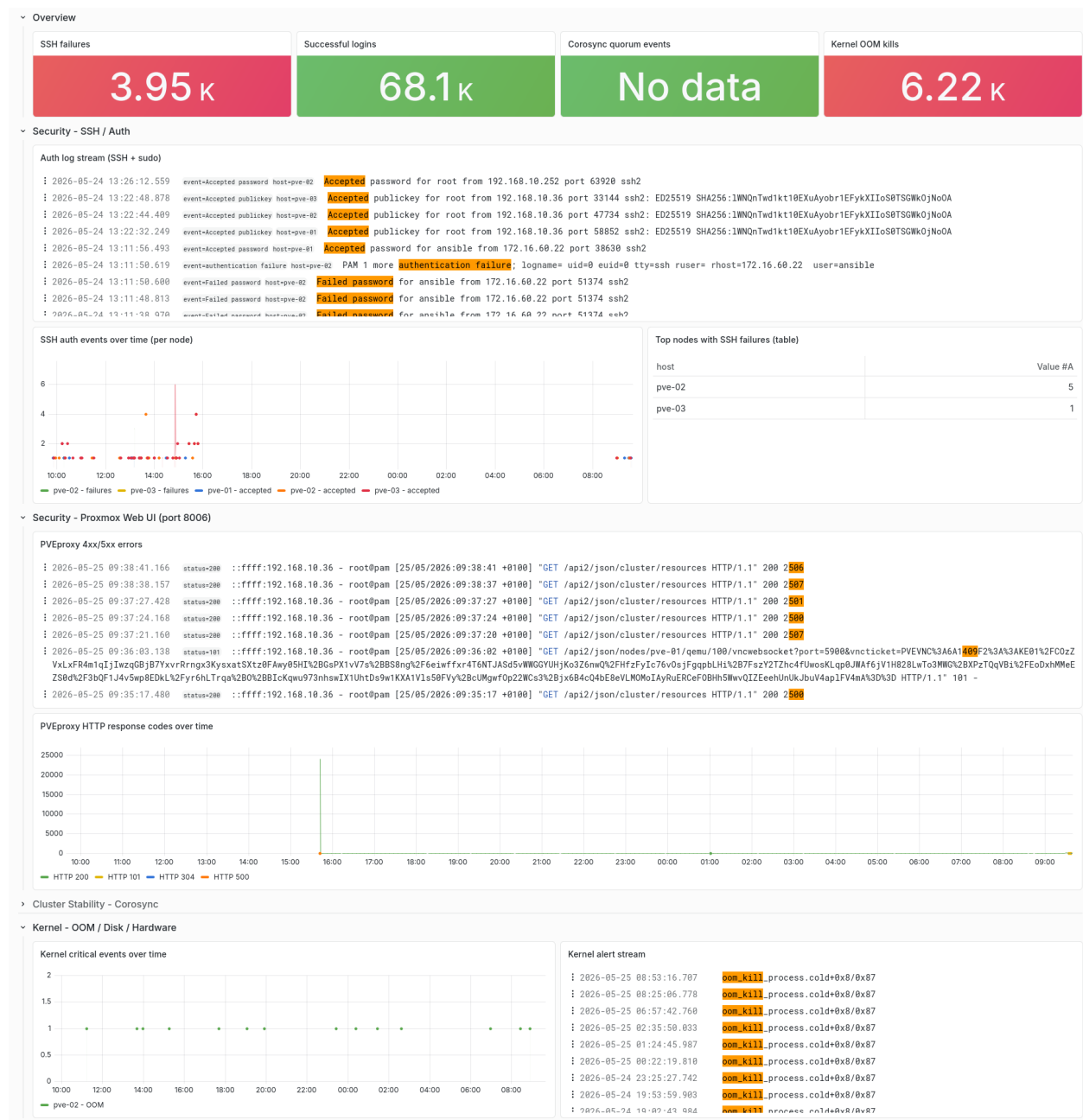
FIGURE IV.62 – Journaux de l’infrastructure visualisés dans Grafana via Loki
