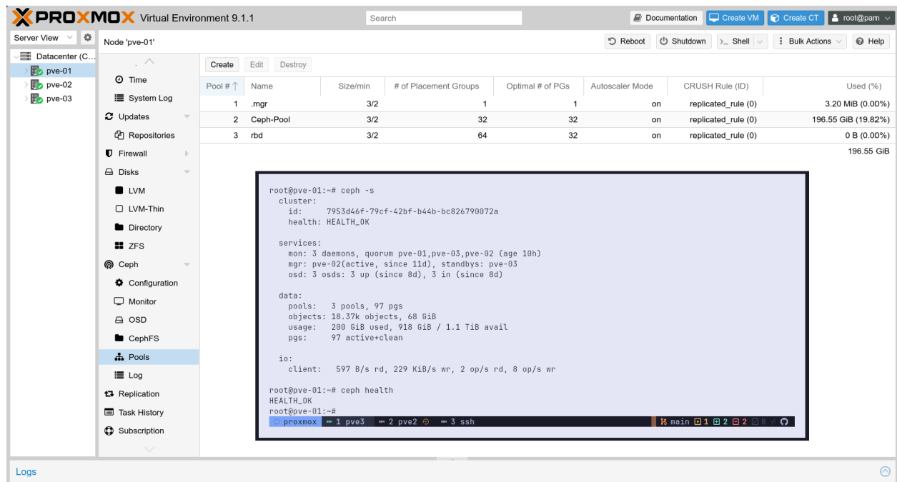
FIGURE IV.39 – État du cluster Ceph montrant le pool RBD
